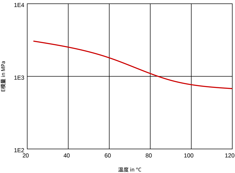
图表 拉伸模量 - 温度
