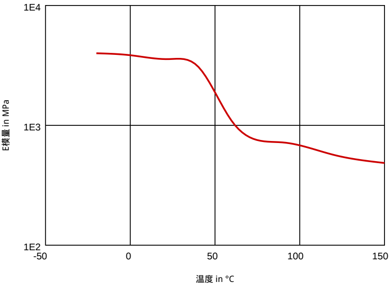
拉伸模量 - 温度 (湿)
