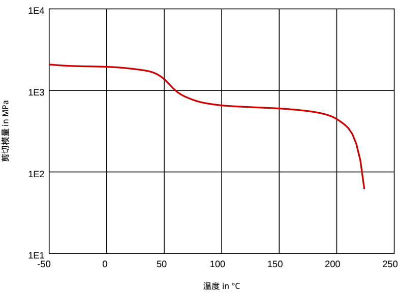
图表 动态剪切模量 - 温度 (干)
